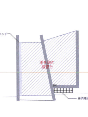
PLAN3(1:150)
