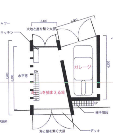
PLAN2(1:150)
