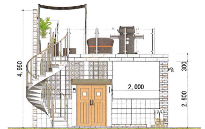
■ 西側立面図 S=1/100 ■
